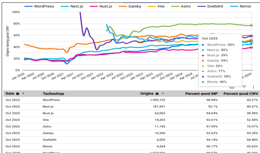
Gambar 3.7 Perbandingan Framework berdasarkan Core Web Vital [45]
